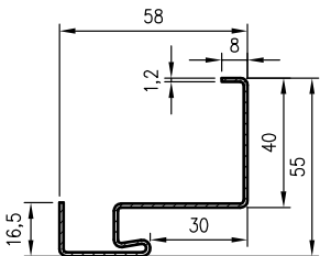
Profil ościezny OSMK
