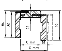
Przekrój TUN z kątem T63
