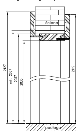
Przekrój pionowy tunelu regulowanego z kątem T80
