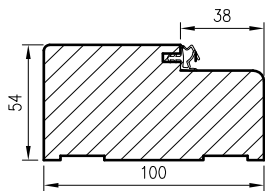
Przekrój ościeżnicy drewnianej do drzwi OLIMP EI60
