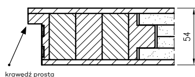
Skrzydło drzwiowe antywłamaniowe - przeciwpożarowe NEFRYT RC3 EI-30
