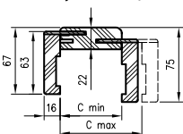
Przekrój TUN z kątem T63
