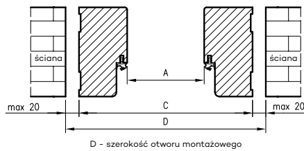
OD OLIMP EI30 do drzwi jednoskrzydłowych
