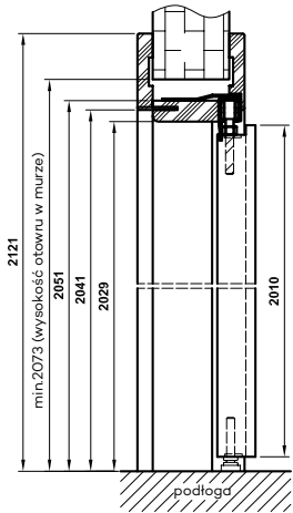
Przekrój pionowy
