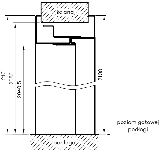
Przekrój pionowy OSRB
