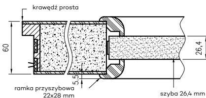
Skrzydło drzwiowe przeciwpożarowe Olimp EI60
