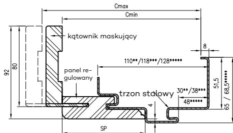
Profil ościeżnicy
