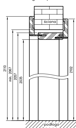
Przekrój pionowy tunelu regulowanego z kątem T63
